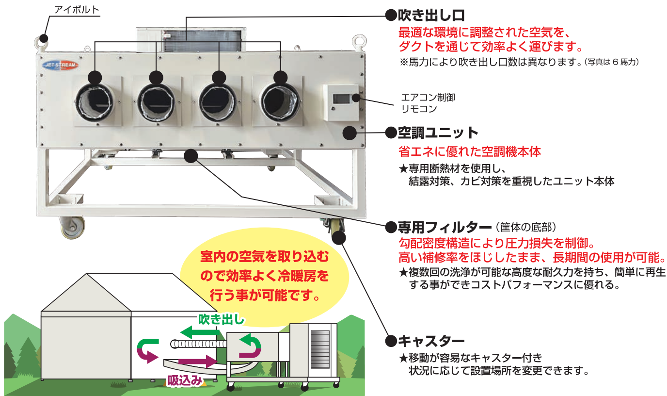
外形図
